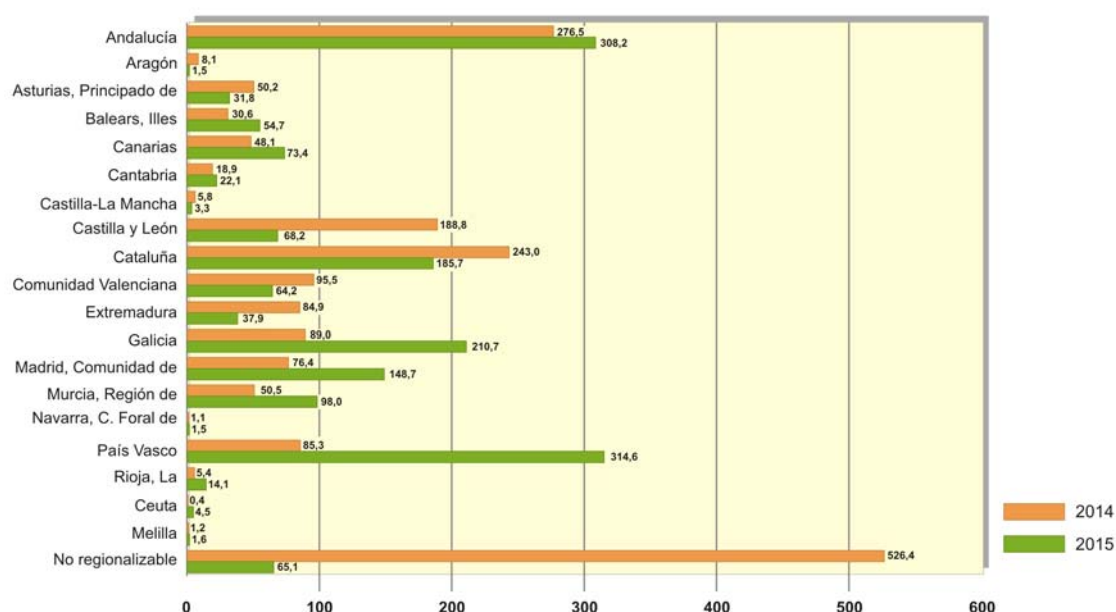
Gráfico 3: Adjudicaciones de obra del Grupo Fomento por Comunidades Autónomas. Años 2014 y 2015 (millones de euros)
