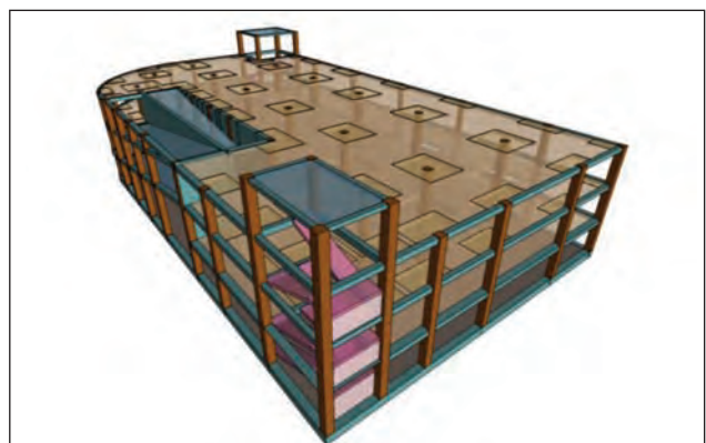
Proyecto de construcción de un aparcamiento en altura en La Manga del Mar Menor
