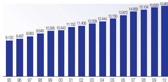
Crecimiento de la red interurbana de vías de gran capacidad (kilómetros)
