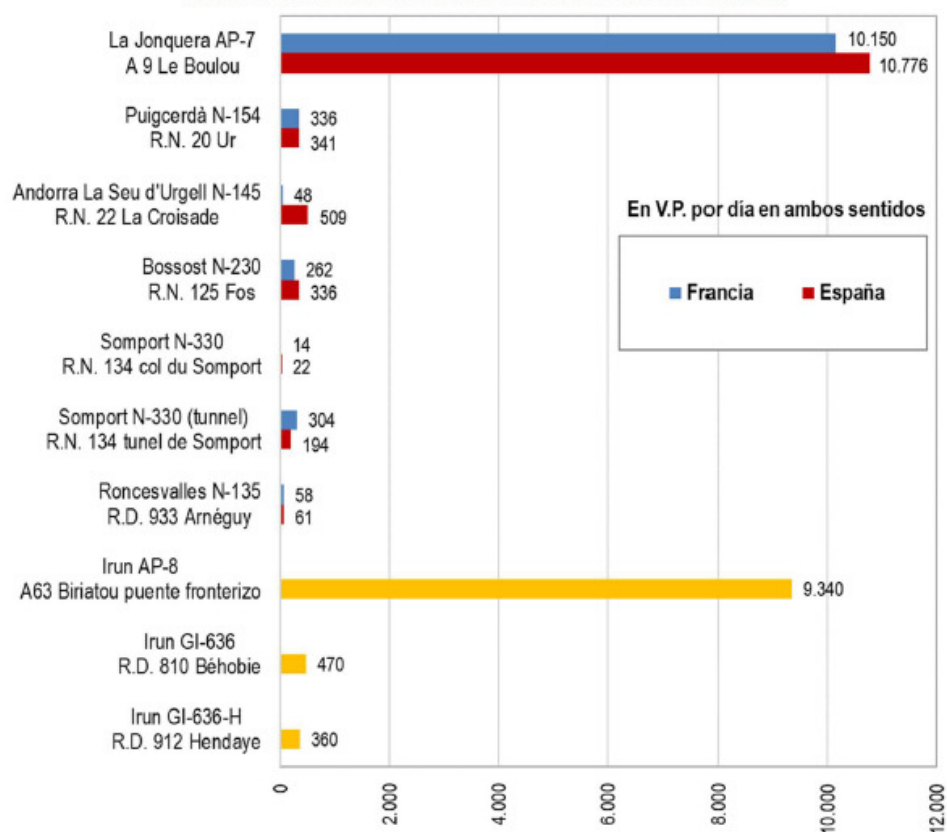
GRÁFICO 28. IMD DE VEHÍCULOS PESADOS (SIN AUTOCARES) EN LOS PUNTOS FRONTERIZOS DE MAYOR TRÁFICO EN 2017
