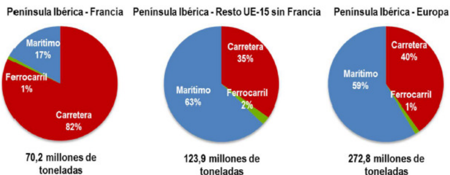
GRÁFICO 35. REPARTO MODAL DEL TRANSPORTE DE MERCANCÍAS A TRAVÉS DE LOS PIRINEOS EN 2017
