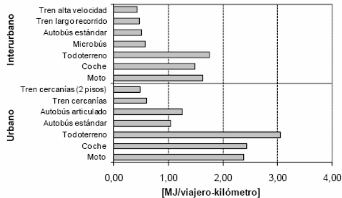
Figura 28: Consumo directo de energía en distintos vehículos de viajeros y tipo de servicio
