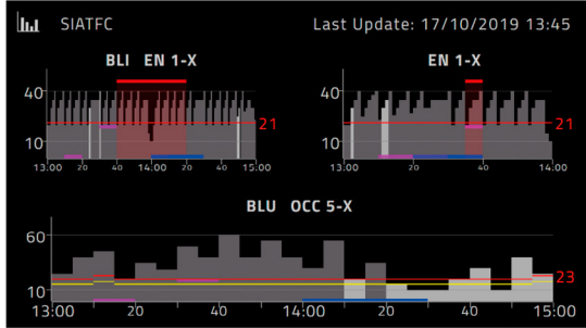
Sistema de Información Auxiliar para controladores aéreos de ENAIRE.
