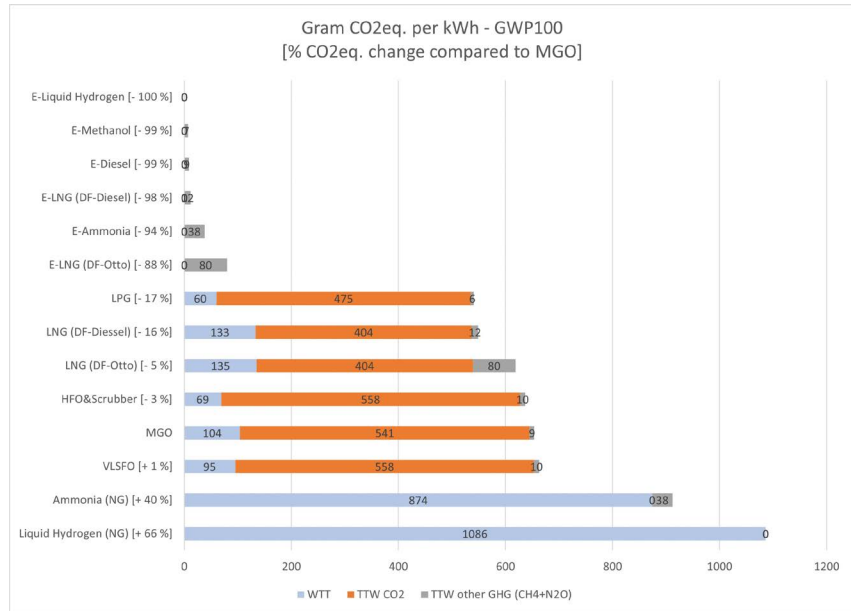
Valores de referencia de los factores de emisión de los combustibles utilizados en el transporte marítimo referidos al factor del gasoil marino (MGO) en gramos de CO 2 /kWh.
