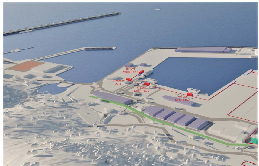
3ª acometida y 3 SET OPS, canalización y tomas para buques ferris y ro-ro. Fuente: Autoridad Portuaria de Bilbao.
