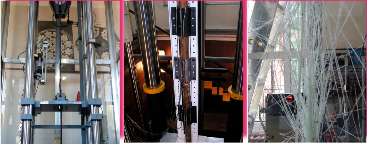
Ensayos mecánicos de aceros de construcción y de armaduras de polímeros reforzados con fibra de vidrio.
