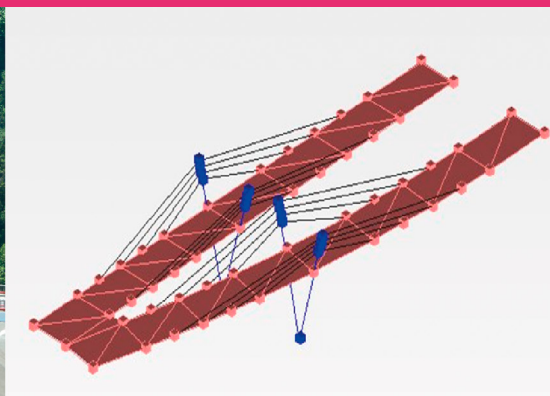
Ensayo dinámico del viaducto de la boca oeste del túnel de Dos Valires (2012).
