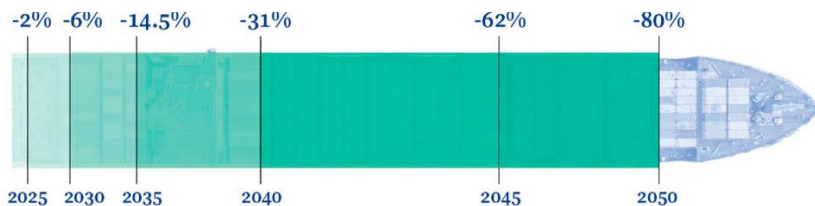
Gráfico de la reducción progresiva de la intensidad de carbono de la energía consumida a bordo.
