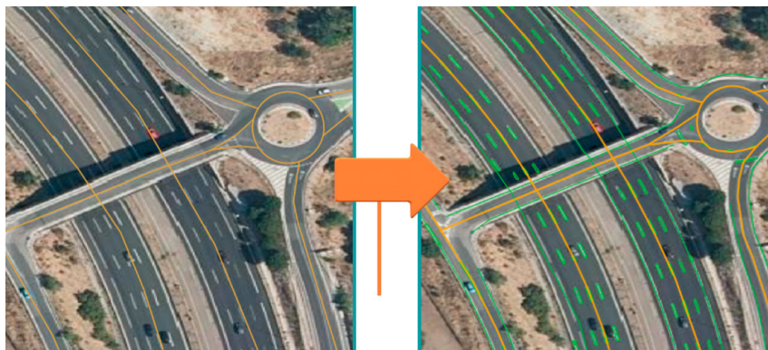
Obtención de las marcas viales a partir de técnicas de Inteligencia Artificial.
