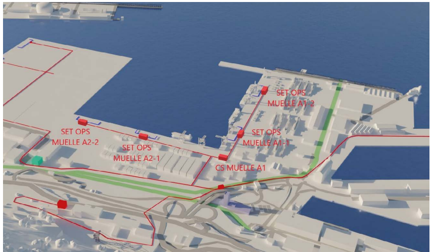
2ª acometida y 4 SET OPS, canalización y tomas para buques portacontenedores. Fuente: Autoridad Portuaria de Bilbao.
