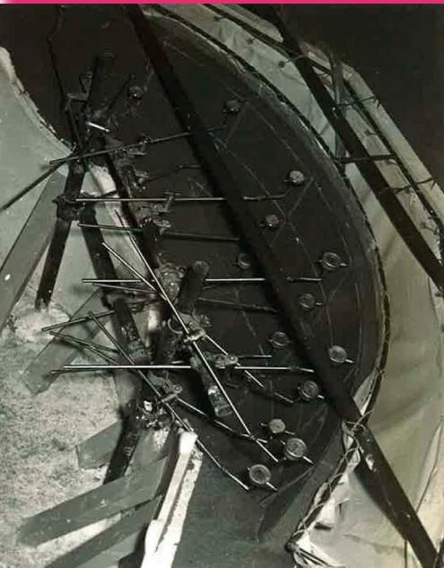
Ensayo del modelo de la presa de Santa Ana (1953).
