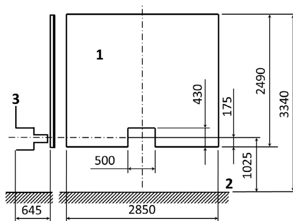
Figura K.1 – Interfaz de vagón con acoplamiento central
