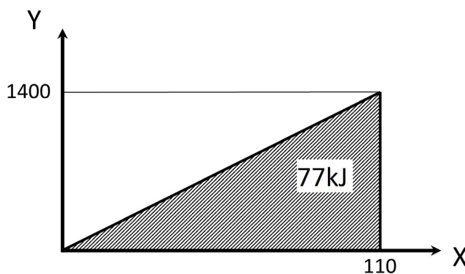
Figura K.2 – Característica del acoplamiento del vagón
