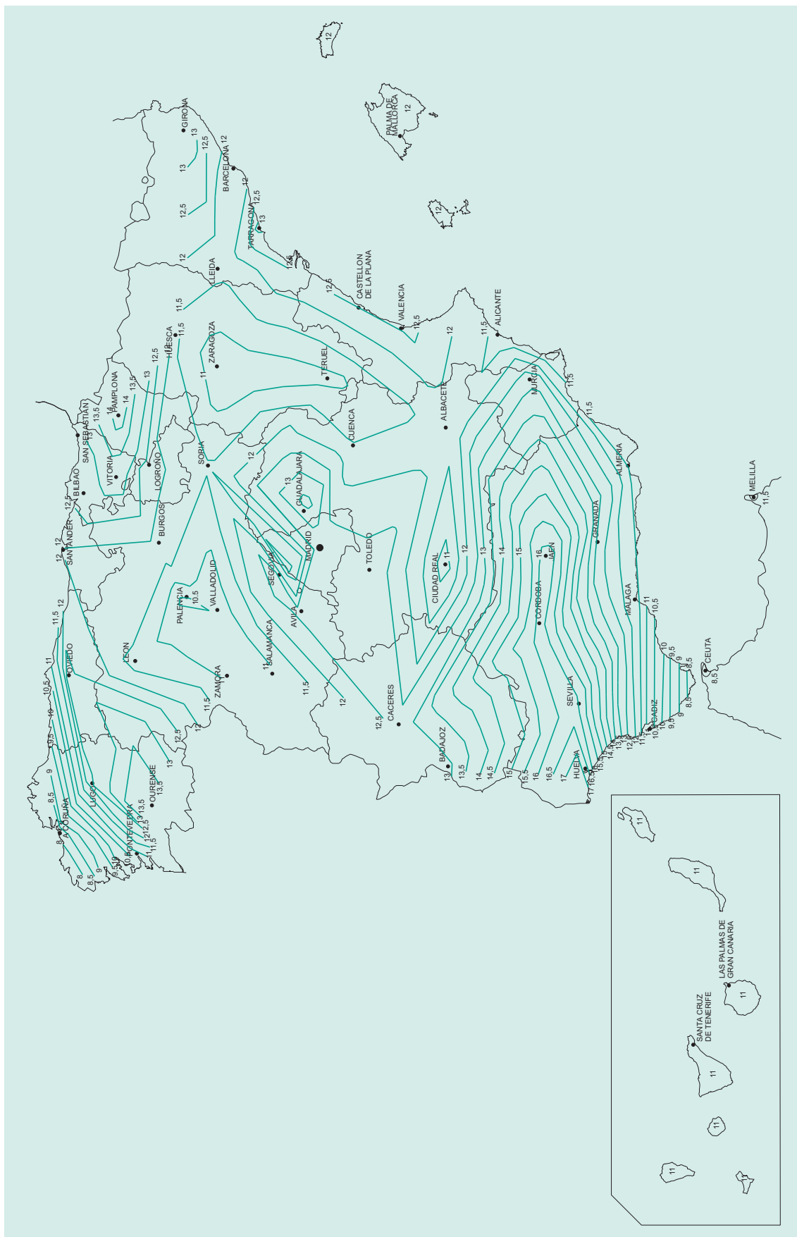
FIGURA 2.26. MAPA DE ISOLÍNEAS PARA LA OBTENCIÓN DE \Delta T_{sl,ref} EN TABLEROS DE LOSAS DE HORMIGÓN.
