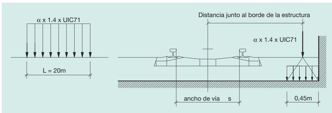
FIGURA 2.37. SITUACIÓN DE PROYECTO II. CARGAS EQUIVALENTES ( Q_{A2d} , q_{A2d} ). (PARA VÍAS SOBRE BALASTO LAS CARGAS PODRÁN DISTRIBUIRSE EN UN ANCHO DE 0,45 m).
