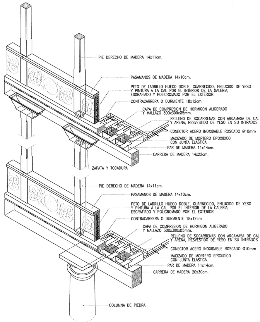
Detalle constructivo de la galería
