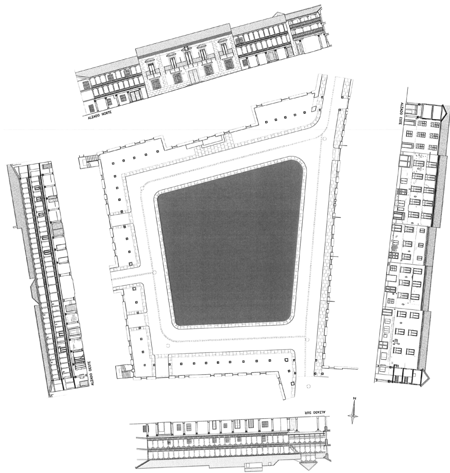
Planta general y alzados
