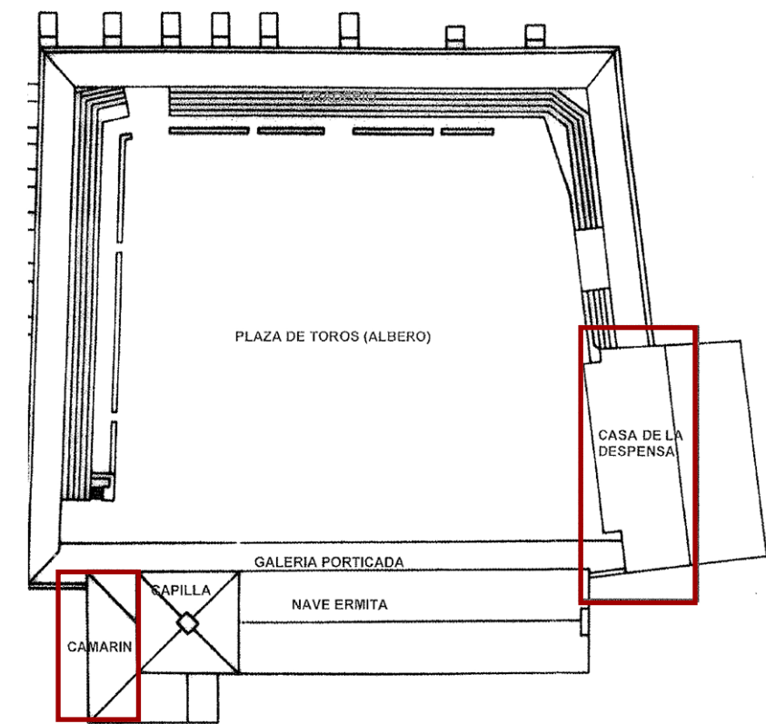
Planta general
